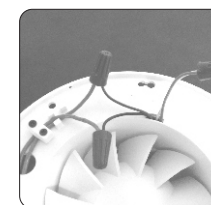
Ligação em 220 Vca
