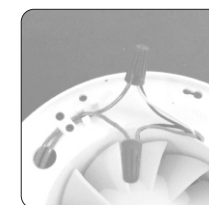
Ligação em 127 Vca
